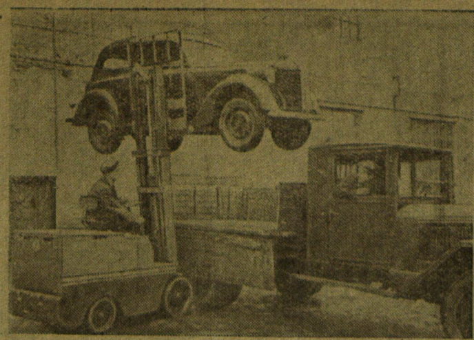
МОСКОВСКИЙ машиностроительный завод имени Орджоникидзе выпустил первую опытную партию автопогрузчиков. Это — новая машина, заменяющая ручной труд на погрузке и выгрузке. Она обладает большой маневренностью. Ее можно использовать для работы в товарном вагоне, в трюме парохода. В ближайшее время предприятие приступит к серийному производству автопогрузчиков. На снимке: автопогрузчик грузит малолитражный автомобиль.
